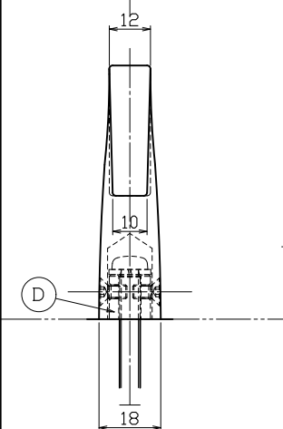
A矢視断面図
