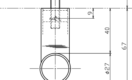
A矢視図
